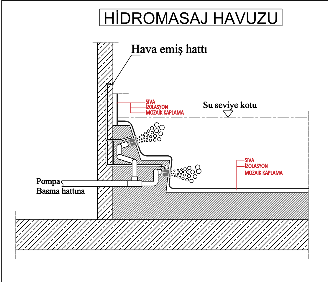
BETONARME MASAJ SİSTEMİ DETAYI
