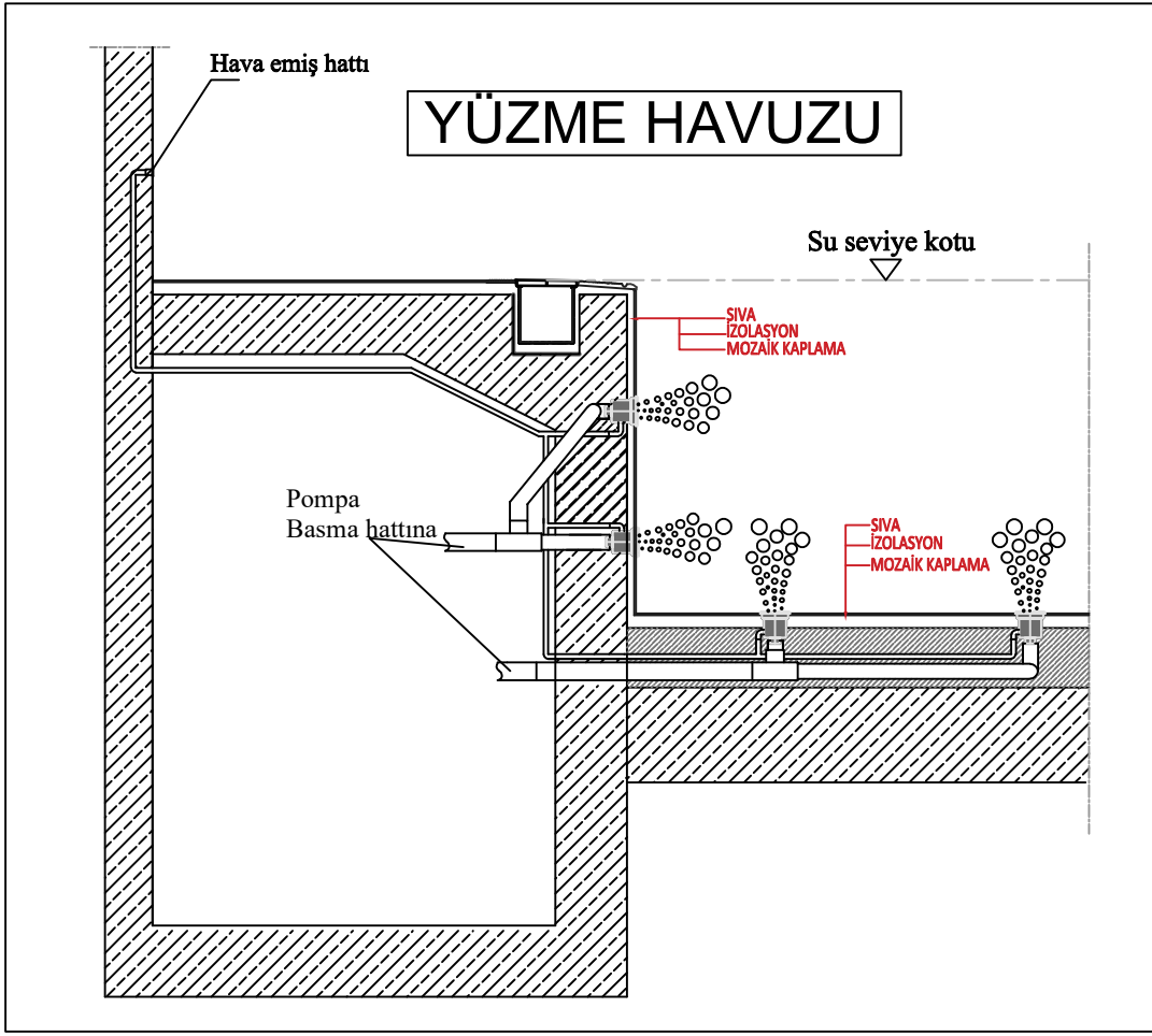
DUVAR VE ZEMİN MASAJ SİSTEMİ DETAYI
